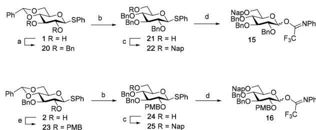
Scheme 4 Synthesis of donor 15 and 16 . (a) BnBr, NaH, DMF, 20 : 96%. (b) \text{BH}_3 ·THF, Cu(OTf) 2 , 21 : 80%; 24 : 76%. (c) NapBr, NaH, DMF, 22 : 91%; 25 : 93%. (d) 1) NIS, acetone : \text{H}_2\text{O} = 10 : 1 (v : v); 2) 2,2,2-trifluoro- N -phenylacetimidoyl chloride, \text{Cs}_2\text{CO}_3 , acetone, yield 15 : 86%; 16 : 84%. (e) PMBCl, NaH, DMF, 94%.
