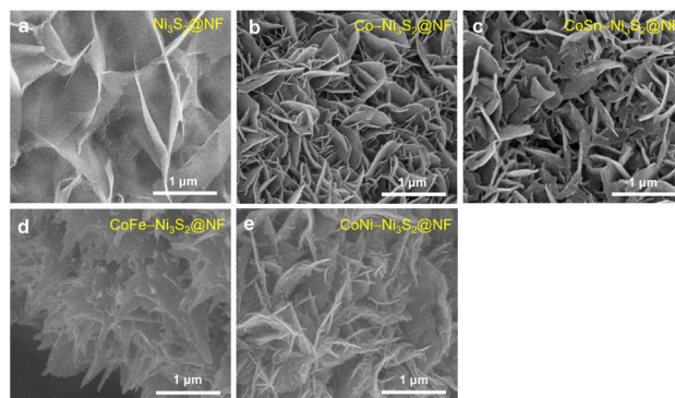
Fig. 2 FE-SEM image of pristine and doped- \text{Ni}_3\text{S}_2\text{@NF} catalysts. (a) \text{Ni}_3\text{S}_2\text{@NF} , (b) \text{Co-Ni}_3\text{S}_2\text{@NF} , (c) \text{CoSn-Ni}_3\text{S}_2\text{@NF} , (d) \text{CoFe-Ni}_3\text{S}_2\text{@NF} , and (e) \text{CoNi-Ni}_3\text{S}_2\text{@NF} .
