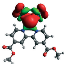
HOMO
