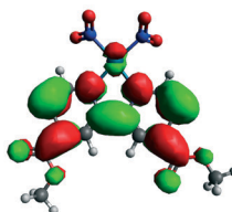
LUMO
