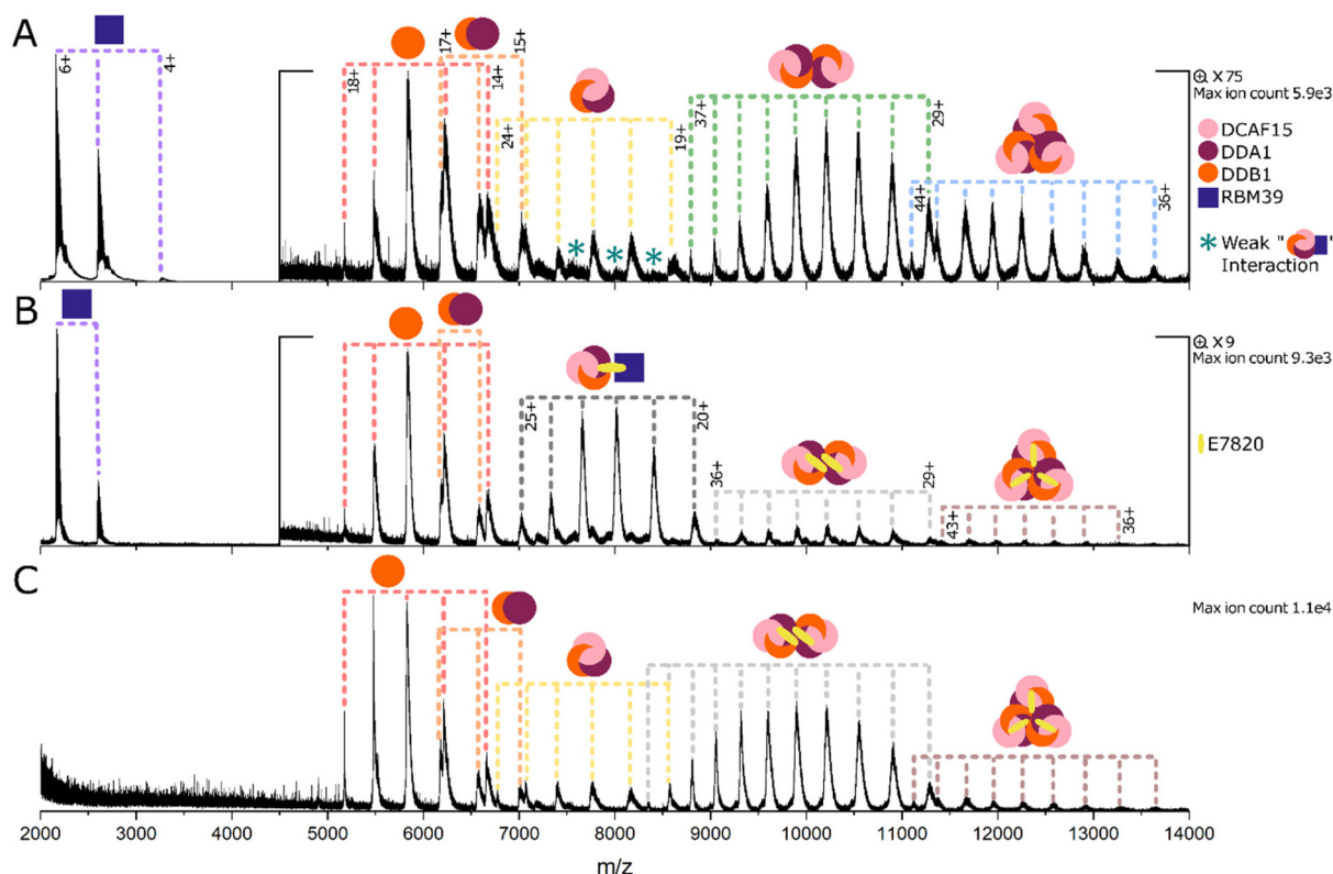
Fig. 3 (A) RBM39 + DCAF15 complex (DCF15 : DDA1 : DDB1). (B) RBM39 + DCAF15 complex + E7820. (C) DCAF15 complex + E7820. Protein concentrations are 5 \mu M and E7820 is 100 \mu M when present. Measured masses of the labelled species are as follows: RBM39 12 978.0 Da. DDB1 93 247 Da. DDA1 : DDB1 104 948 Da. DCAF15 complex (monomer) 162 392 Da. DCAF15 complex (dimer) 324 792 Da. DCAF15 complex (trimer) 487 208 Da. Ternary complex 175 725 Da. DCAF15 complex (dimer) + 2xE7820 325 463 Da. DCAF15 complex (trimer) + 3xE7820 488 219 Da. Masses given to the nearest 1 Da, and further details are given in Table S3.†
