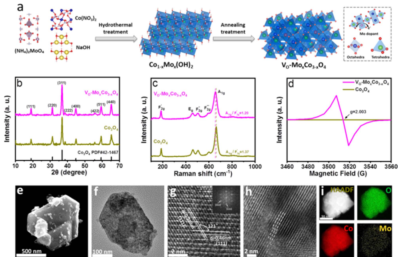
Fig. 1 (a) Scheme of the synthetic process for V_O-Mo_xCo_{3-x}O_4 . (b) XRD patterns of V_O-Mo_xCo_{3-x}O_4 and Co_3O_4 . (c) Raman spectra of V_O-Mo_xCo_{3-x}O_4 and Co_3O_4 . (d) EPR spectra of V_O-Mo_xCo_{3-x}O_4 and Co_3O_4 . (e) SEM image of V_O-Mo_xCo_{3-x}O_4 . (f-h) TEM images of V_O-Mo_xCo_{3-x}O_4 . (i) HAADF-STEM and corresponding elemental mapping images of V_O-Mo_xCo_{3-x}O_4 .
