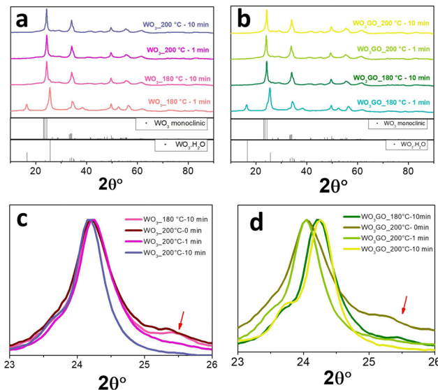
Fig. 4 XRD of (a) WO 3 _180 °C-1 min, WO 3 _180 °C-10 min, WO 3 _200 °C-1 min, WO 3 _200 °C-10 min and (b) WO 3 GO_180 °C-1 min, WO 3 GO_180 °C-10 min, WO 3 GO_200 °C-1 min and WO 3 GO_200 °C-10 min. Magnified XRD region between 23 and 26° of (c) WO 3 _180 °C-10 min, WO 3 _200 °C-0 min, WO 3 _200 °C-1 min, WO 3 _200 °C-10 min and (d) WO 3 GO_180 °C-10 min, WO 3 GO_200 °C-0 min, WO 3 GO_200 °C-1 min and WO 3 GO_200 °C-10 min.
