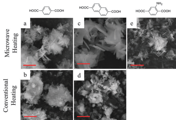
Fig. 2 SEM images of (a) MIL-140A-MW, (b) MIL-140A-CE, (c) MIL-140B-MW, (d) MIL-140B-CE and (e) MIL-140A-NH 2 -MW (scale bar = 3 μm).
