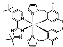
Ir(dfb-pz) 2 (bbptz) 53
