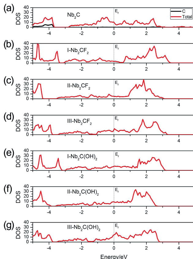
Fig. 2 Total DOS of (a) \text{Nb}_2\text{C} , (b) I- \text{Nb}_2\text{CF}_2 , (c) II- \text{Nb}_2\text{CF}_2 , (d) III- \text{Nb}_2\text{CF}_2 , (e) I- \text{Nb}_2\text{C(OH)}_2 , (f) II- \text{Nb}_2\text{C(OH)}_2 and (g) III- \text{Nb}_2\text{C(OH)}_2 . The Fermi levels are set to zero.
