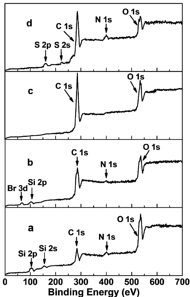
Fig. 2 XPS survey spectra of \text{NH}_2@SiO_2 (a), \text{Br}@SiO_2 (b), \text{PGMA}@SiO_2 (c) and \text{DTC-PGMA}@SiO_2 (d) samples.
