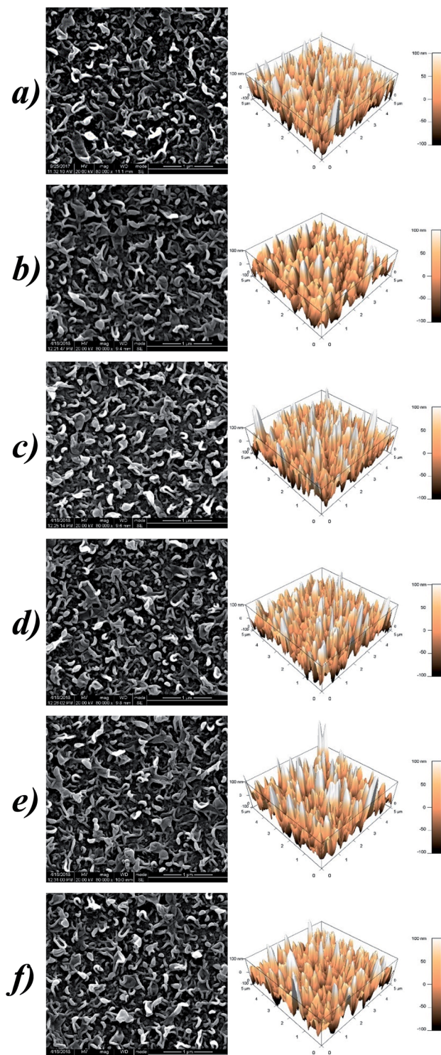
Fig. 5 SEM and AFM images of (a) L-0; (b) L-1; (c) L-3; (d) L-5; (e) L-7; and (f) L-10.
