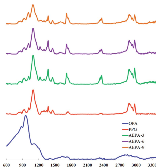
Fig. 2 FTIR spectra.
