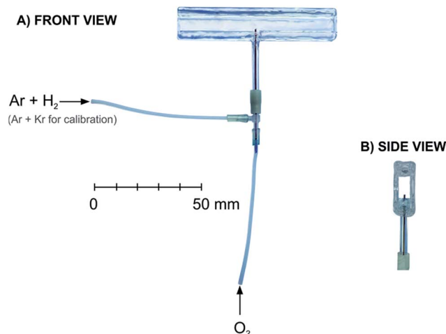
Fig. 2 Atomizer.
