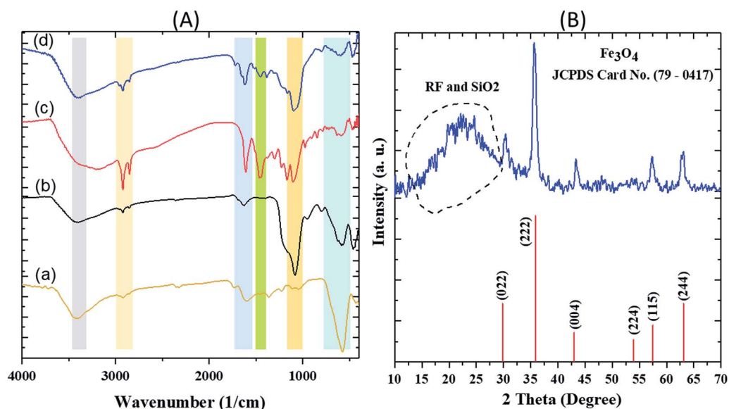
Fig. 2 FT-IR spectra of (A) (a) \text{Fe}_3\text{O}_4 (b) \text{Fe}_3\text{O}_4@/\text{SiO}_2 (c) \text{Fe}_3\text{O}_4@/\text{SiO}_2@/\text{RF} and (d) \text{Fe}_3\text{O}_4@/\text{SiO}_2@/\text{RF-SO}_3\text{H} and (B) XRD pattern of \text{Fe}_3\text{O}_4@/\text{SiO}_2@/\text{RF-SO}_3\text{H} sample.
