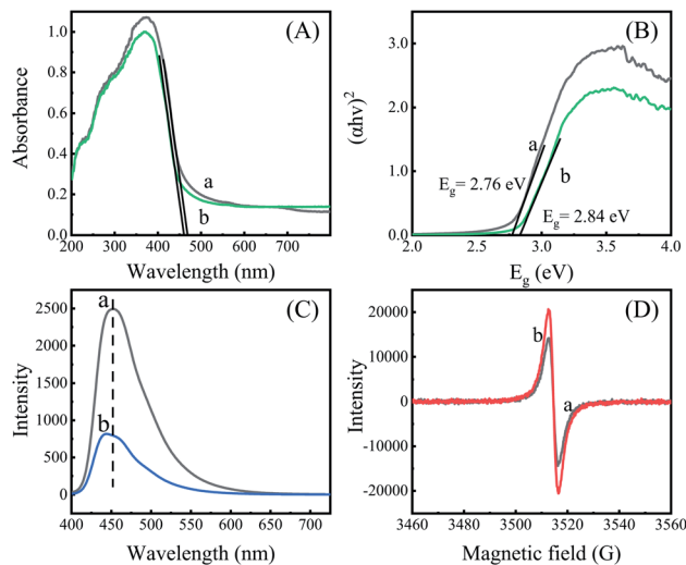
Fig. 5 (A) Solid diffuse reflectance spectra; (B) Tauc plots; (C) fluorescence spectra, \lambda_{\text{ex}} = 380 \text{ nm} ; (D) EPR spectra. (a) g\text{-C}_3\text{N}_4 , (b) g\text{-C}_3\text{N}_4\text{-Sr}_2\text{V}_2\text{O}_7 .
