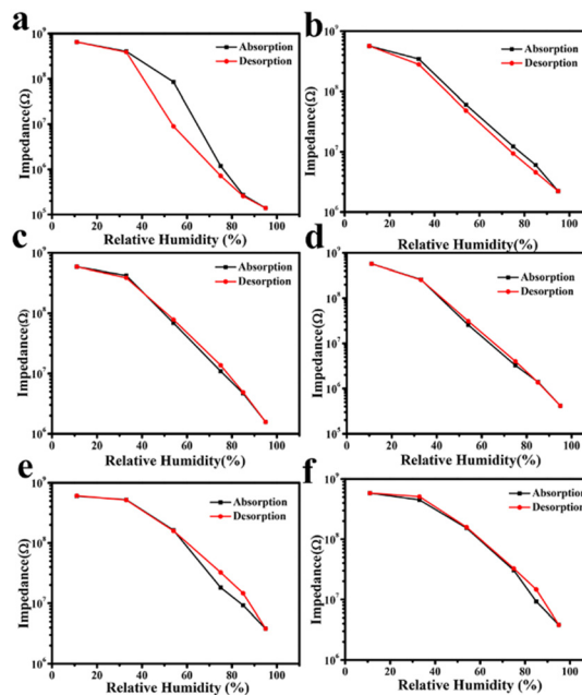
Fig. 7 Humidity hysteresis of sensors based on (a) ZrO 2 , (b) C–N/ZrO 2 -1, (c) C–N/ZrO 2 -2, (d) C–N/ZrO 2 -3, (e) C–N/ZrO 2 -4 and (f) C–N/ZrO 2 -5.
