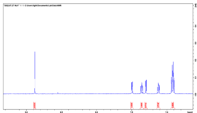
Fig. 5 ^1\text{H} NMR spectra of \text{MJ}_1 .
