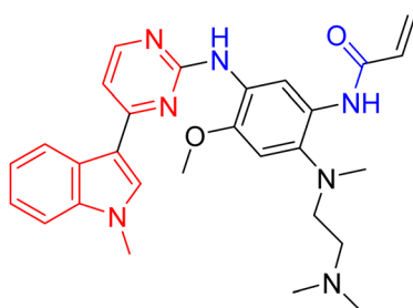
Osimertinib
