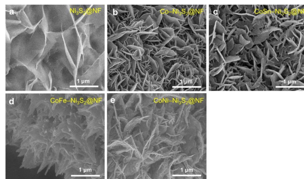
Fig. 2 FE-SEM image of pristine and doped- \text{Ni}_3\text{S}_2@\text{NF} catalysts. (a) \text{Ni}_3\text{S}_2@\text{NF} , (b) \text{Co-Ni}_3\text{S}_2@\text{NF} , (c) \text{CoSn-Ni}_3\text{S}_2@\text{NF} , (d) \text{CoFe-Ni}_3\text{S}_2@\text{NF} , and (e) \text{CoNi-Ni}_3\text{S}_2@\text{NF} .
