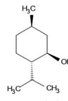
Menthol
