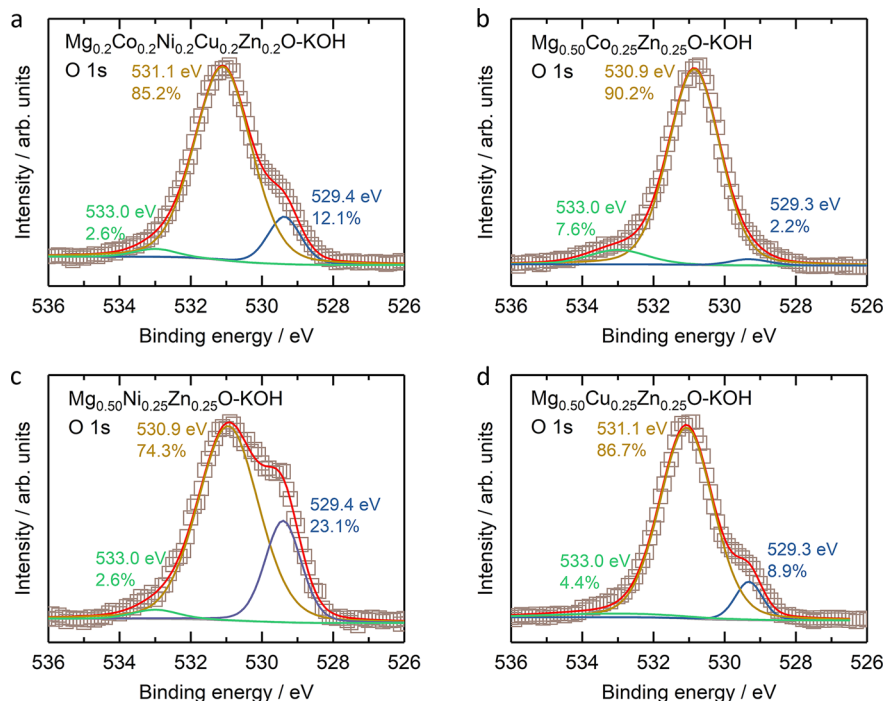
Fig. 8 The O 1s XPS results of (a) Mg 0.2 Co 0.2 Ni 0.2 Cu 0.2 Zn 0.2 O, (b) Mg 0.50 Co 0.25 Zn 0.25 O, (c) Mg 0.50 Ni 0.25 Zn 0.25 O, and (d) Mg 0.50 Cu 0.25 Zn 0.25 O.
