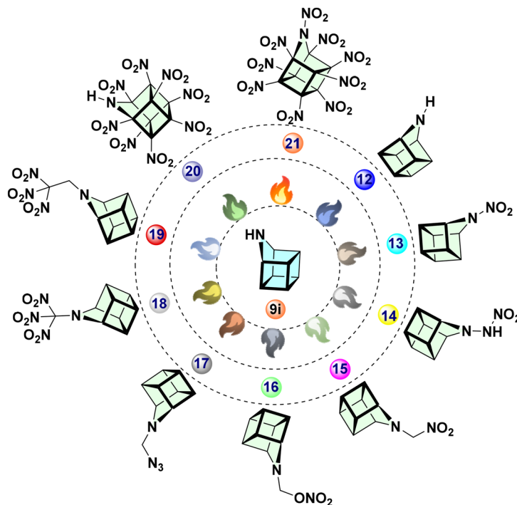
9-Azapentacyclo[4.3.0.0 2,5 .0 3,8 .0 4,7 ]nonane ( 12 ). 9-Nitro-9-azapentacyclo[4.3.0.0 2,5 .0 3,8 .0 4,7 ]nonane ( 13 ). 9-Azapentacyclo[4.3.0.0 2,5 .0 3,8 .0 4,7 ]nonan-9-yl]nitramide ( 14 ). N-9-(Nitromethyl)-9-azapentacyclo[4.3.0.0 2,5 .0 3,8 .0 4,7 ]nonane ( 15 ). 9-Azapentacyclo[4.3.0.0 2,5 .0 3,8 .0 4,7 ]nonan-9-yl]methyl nitrate ( 16 ). 9-(Azidomethyl)-9-azapentacyclo[4.3.0.0 2,5 .0 3,8 .0 4,7 ]nonane ( 17 ). 9-(Trinitromethyl)-9-azapentacyclo[4.3.0.0 2,5 .0 3,8 .0 4,7 ]nonane ( 18 ). 9-(2,2,2-Trinitroethyl)-9-azapentacyclo[4.3.0.0 2,5 .0 3,8 .0 4,7 ]nonane ( 19 ). 1,2,3,4,5,6,7,8-Octanitro-9-azapentacyclo[4.3.0.0 2,5 .0 3,8 .0 4,7 ]nonane ( 20 ). 1,2,3,4,5,6,7,8,9-Nonanitro-9-azapentacyclo[4.3.0.0 2,5 .0 3,8 .0 4,7 ]nonane ( 21 ).
