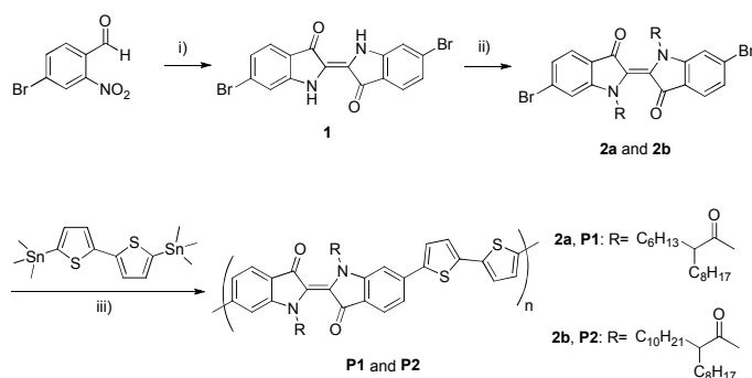
Scheme 1. Synthetic route to indigo monomers 2a and 2b and polymers P1 and P2 : i) NaOH/acetone/r.t.; ii) a) NaH/NMP/r.t., b) RCOCl/r.t.; iii) Pd 2 (dba) 3 /P(o-tolyl) 3 /chlorobenzene/90 °C.
