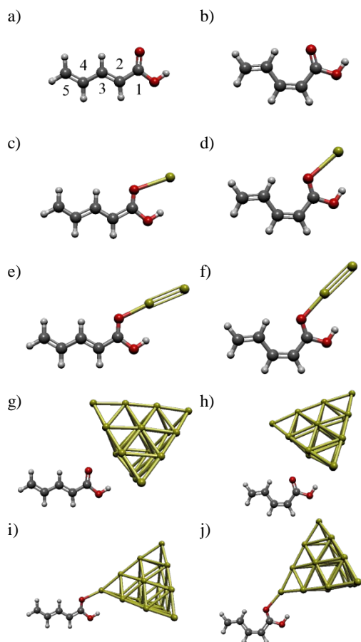
Figure 1. The systems under study: a) trans -PDA b) cis -PDA c) trans -PDA-Au d) cis -PDA-Au e) trans -PDA-Au 2 f) cis -PDA-Au 2 g) trans -PDA-Au 20 surface h) cis -PDA-Au 20 surface i) trans -PDA-Au 20 vertex j) cis -PDA-Au 20 vertex.
