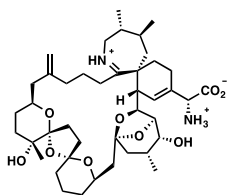
pinnatoxin C
