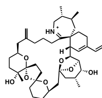
pinnatoxin G
