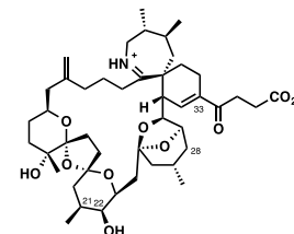
pinnatoxin D
