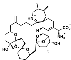
pinnatoxin B
