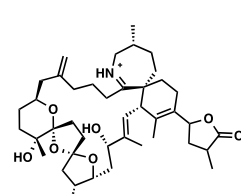
spirolide B
