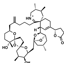
pinnatoxin F
