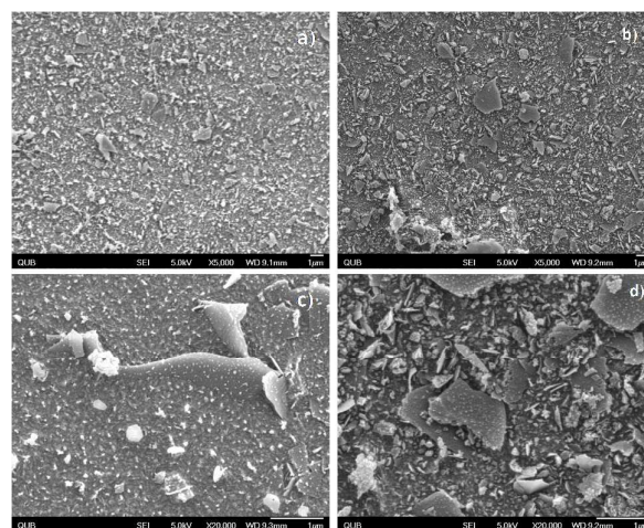
Fig. 2- FESEM images of PA6/GNPs nanocomposites after plasma etching process: a) PA6/10%C500-50rpmx5K, b) PA6/20%C500-200rpmx5K, c) PA6/10%M5-50rpmx20K and d) PA6/20%C500-200rpmx20K.
