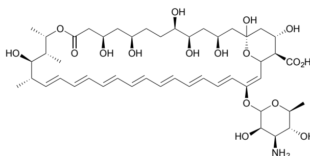
Figure 1. Structure of AmB
