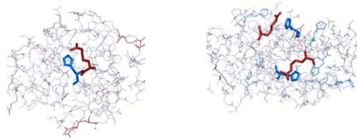
Lysozyme C ( 5c )
