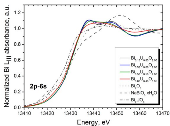
Fig. 4.a Bi L_{III} XANES spectra of Bi_{0.15}U_{0.85}O_{2.00} , Bi_{0.32}U_{0.68}O_{2.00} , Bi_{0.50}U_{0.50}O_{2.00} , and Bi_{0.60}U_{0.40}O_{1.95} .
