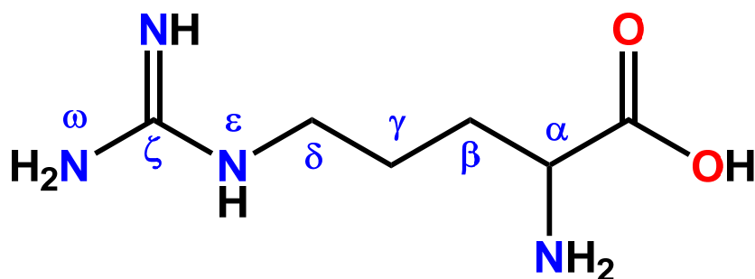
Arginine ( C_6H_{14}N_4O_2 )
