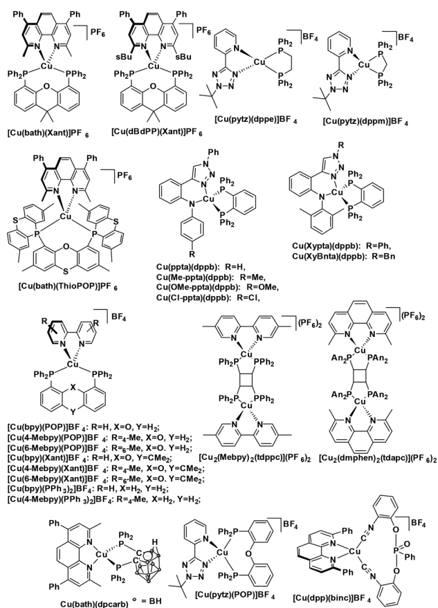
Fig. 6 [Cu(N Δ N)(P Δ P)] + and [Cu(N Δ N')(P Δ P)] type complexes.
