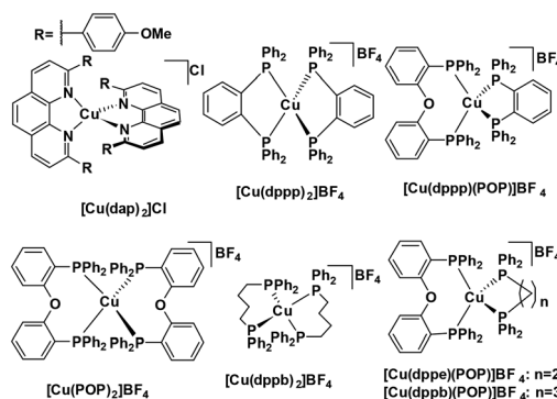
Fig. 7 [Cu(N Δ N) 2 ] + and [Cu(P Δ P) 2 ] + complexes.
