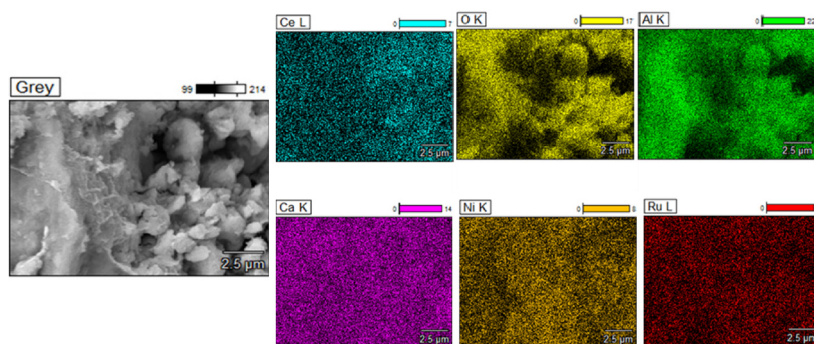
Fig. 13 SEM and EDX mapping of NiRuCa.
