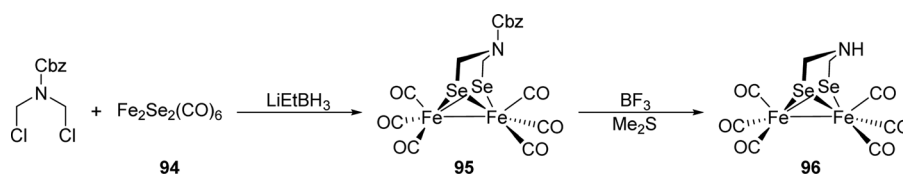
Fig. 34 Synthetic pathway to Fe_2(adSe)(CO)_6 ( 96 ).
