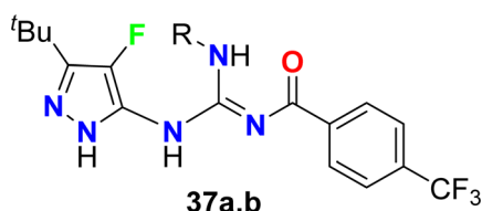
37a: R = 2-Cl-4-FC 6 H 3 , 37b: R = Bu t
