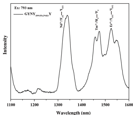
Fig. 2 Downshifting emission spectrum of \text{NaGdF}_4\text{:}49\%\text{Yb}, 1\%\text{Tm}@ \text{NaYF}_4\text{:}20\%\text{Yb}@ \text{NaNdF}_4\text{:}10\%\text{Yb}@ \text{NaYF}_4\text{:}20\%\text{Yb}, 2\%\text{Er}@ \text{NaYF}_4 nanocrystals.
